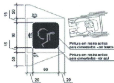
Detalhe das rampas em corte e planta
